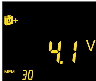
2. Anzeige: Kontaktspannung
